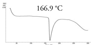
Fig.1. DSC
